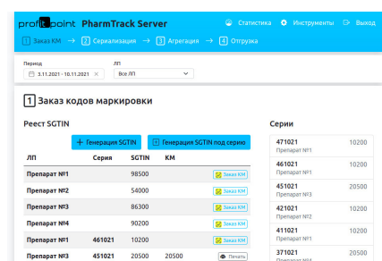
интерфейс серверного ПО
